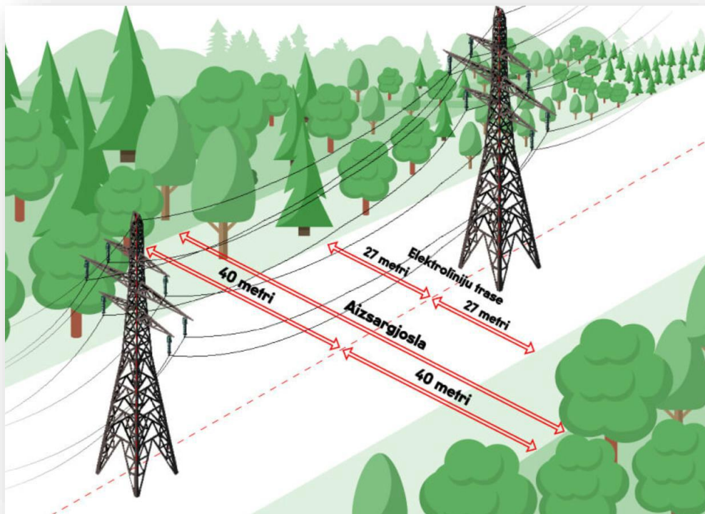
20.att. 330 kV elektrolīnijas trases aizsargjoslas platums
