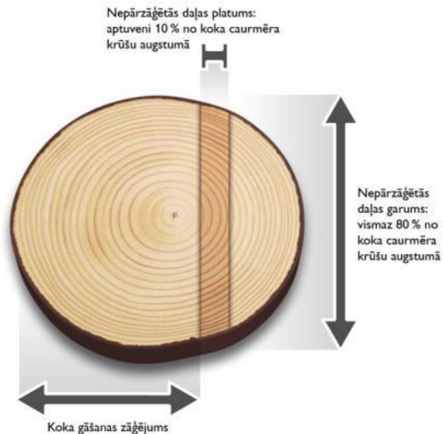
30.att. Koka aizzāģējuma drošības josla
